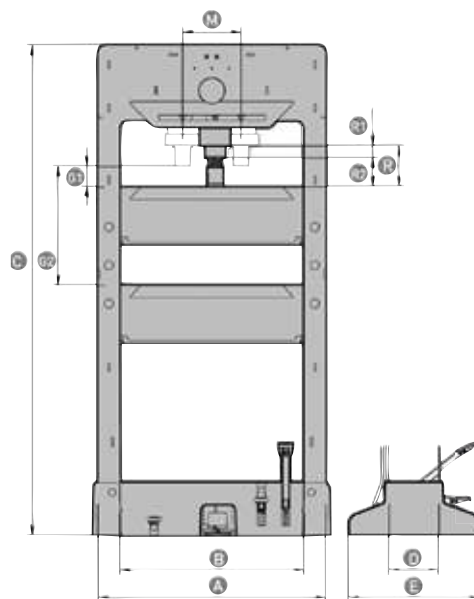
Protection de Presse pour modèle PRC
